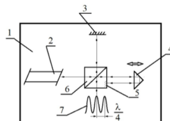
Рисунок 2 – Предлагаемое устройство
